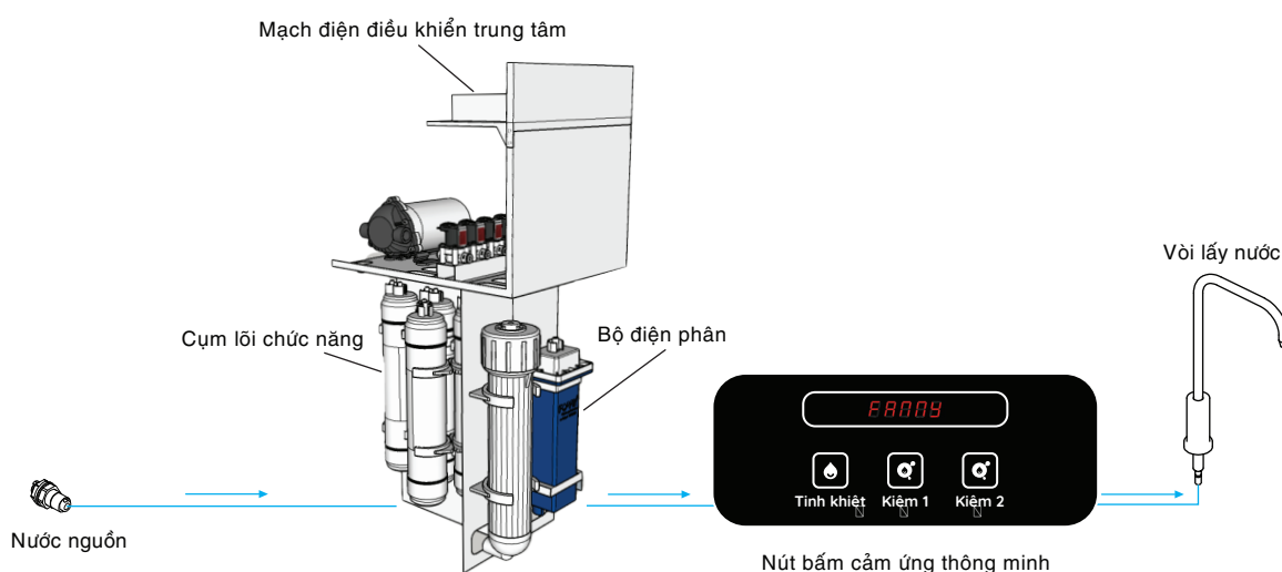
Sơ đồ máy lọc nước RO - Ion kiềm
